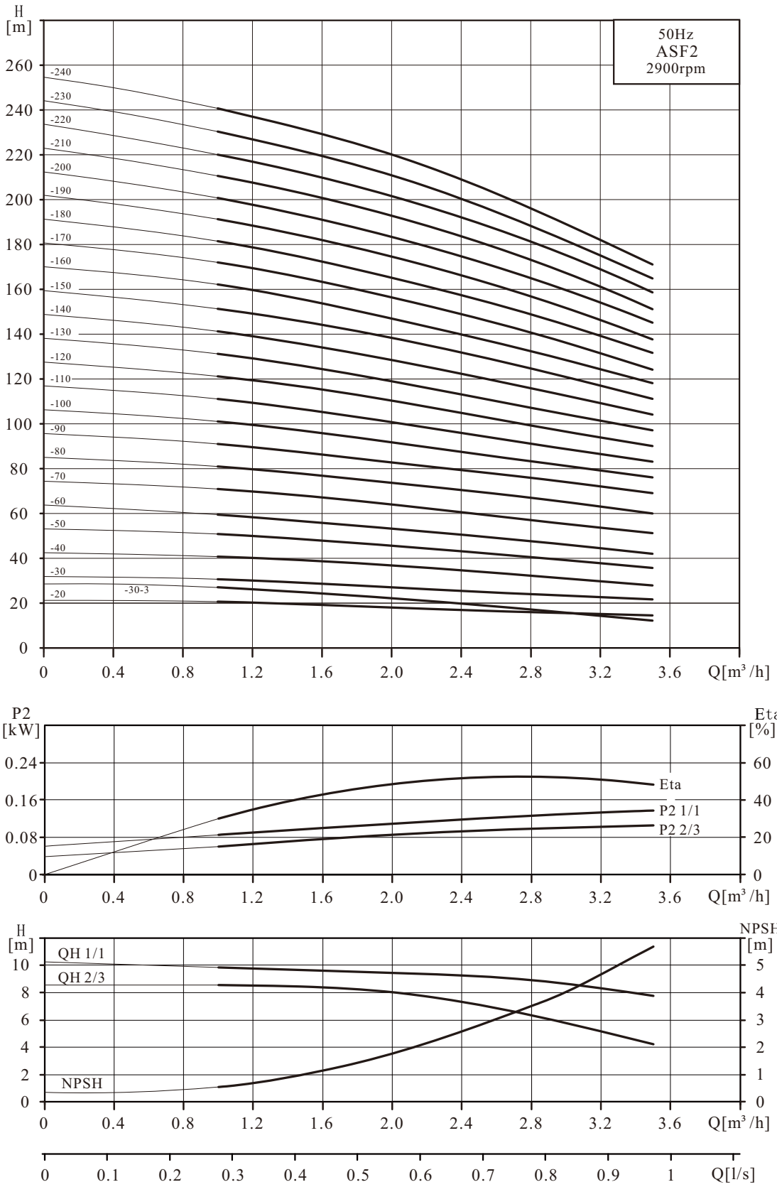
性能曲线
