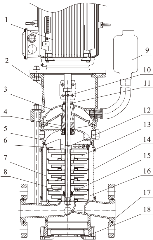
结构图ASF1,2,3,4,5
